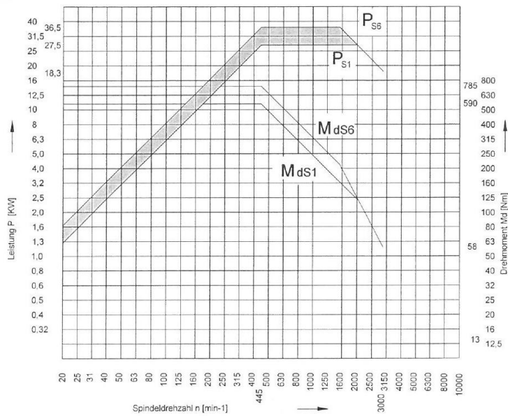
Leistungsdaten NEF 600
