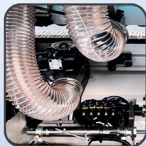
Radiusziehklingenaggregat mit Spänebox
