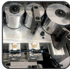
Andruckzone pneumatisch positionierbar
