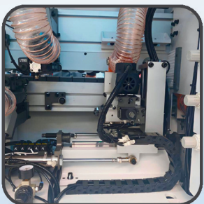
Abrundaggregat
