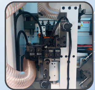
Radiusfräsaggregat mit 2 pneumatischen Positionen
