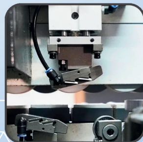
Flachziehklingenaggregat mit Doppelmesser
