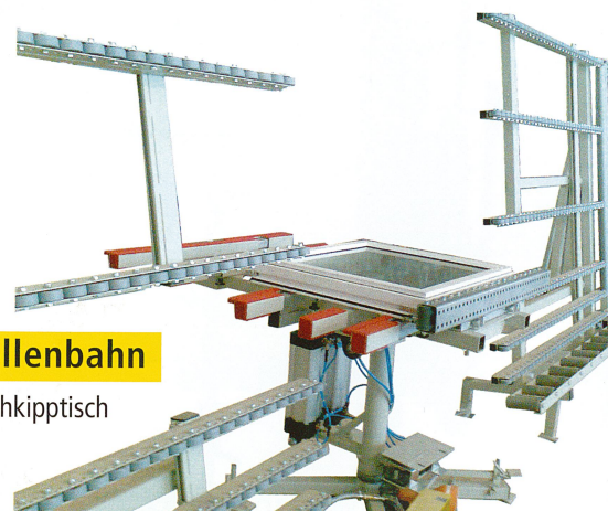
RU-DKFA Dreh-Kipptisch
