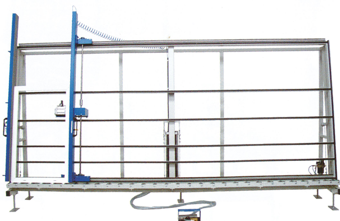
RU-VGP Verglasungs- und Kontrollpresse
