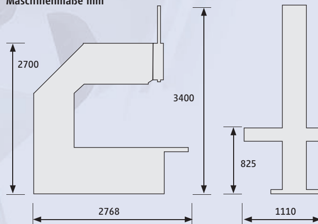
Maschinenmaße mm
