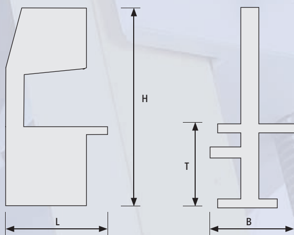
Maschinentischmaße mm
